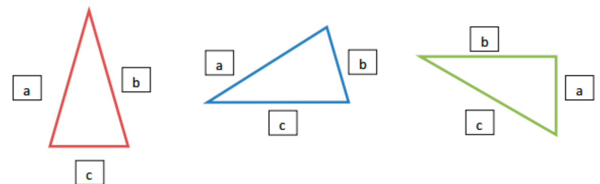
Položaji Jednakokračnog trokuta
